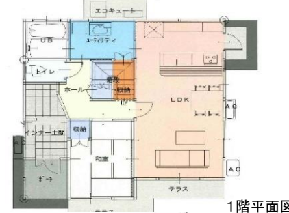
1階平面図
